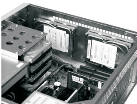
Фото 1. Корзина HDD с установленным держателем корзины на резиновых амортизаторах
