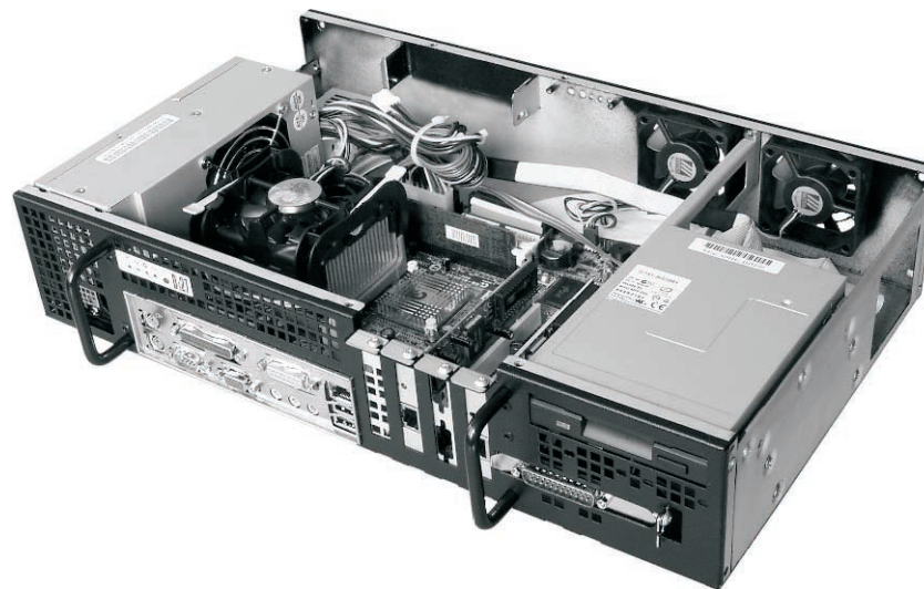
Фото 3. Корпус, подготовленный для крепления в 19" стойке тыльной стороной.
